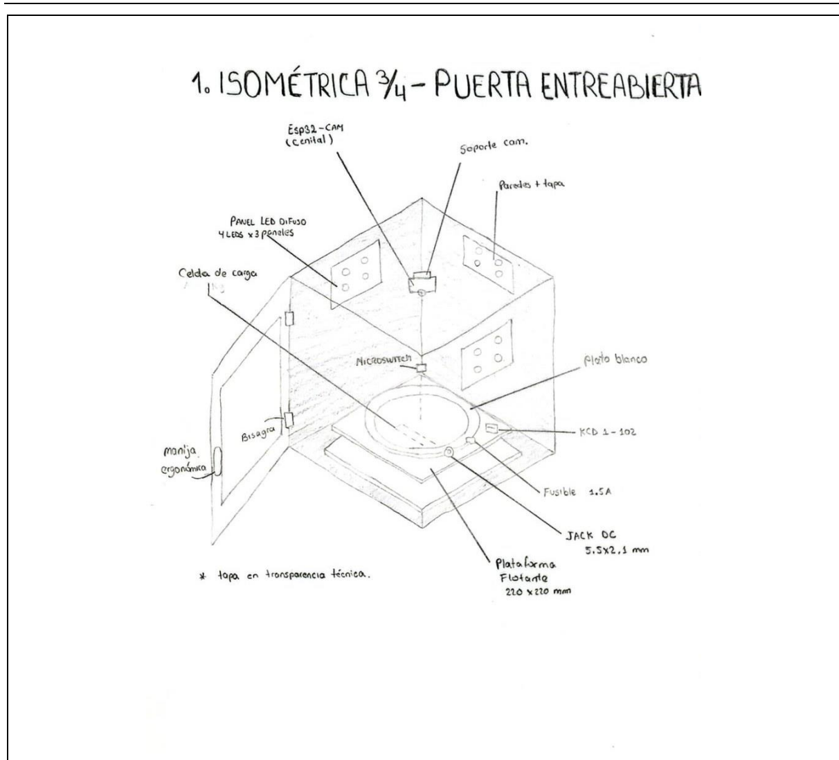
Figura 4: Vista isométrica \frac{3}{4} del Concepto C, con la puerta entreabierta Fuente: Equipo 10
