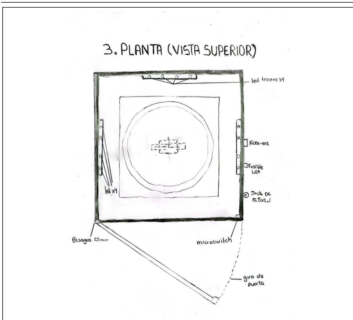
Figura 6: Planta (vista superior) del Concepto C Fuente: Equipo 10
